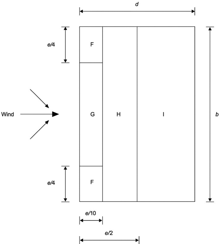
Mit Attika
