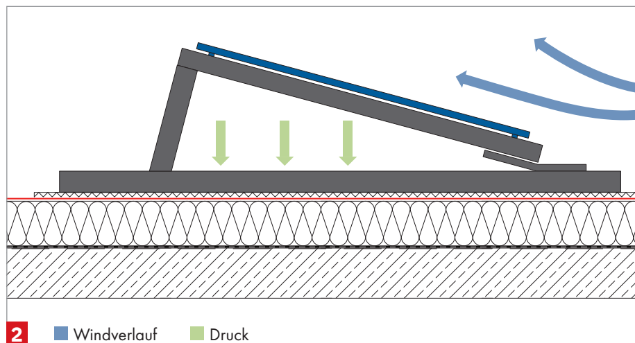
Abbildung 2: Aerodynamisches System
