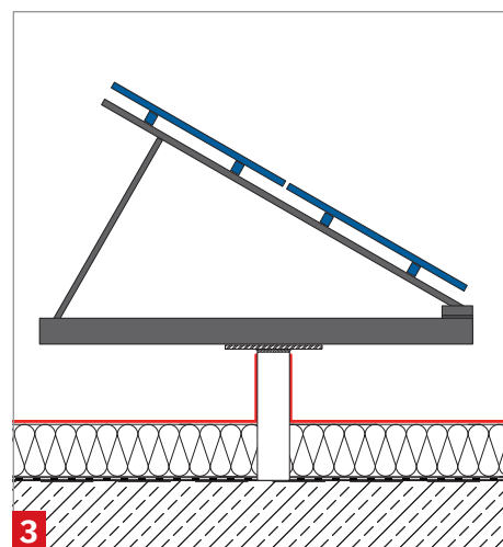
Abbildung 3: Aufgeständertes System
