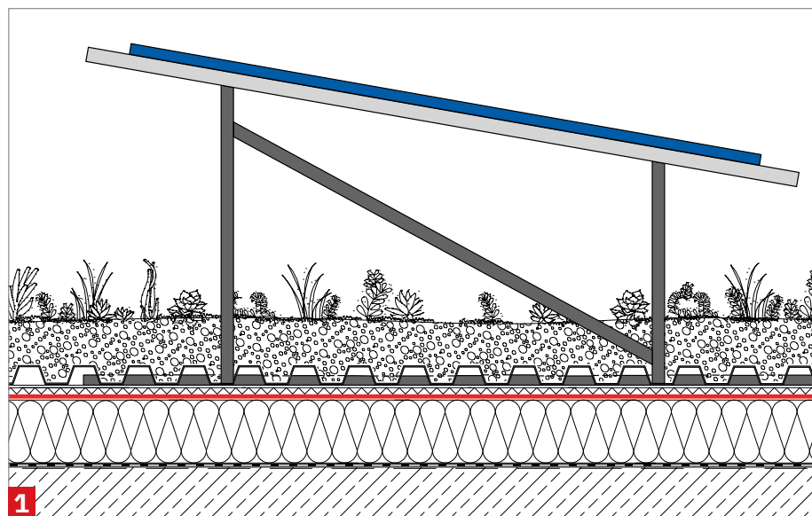
Abbildung 1: Solar-ballastiertes System-Gründach
